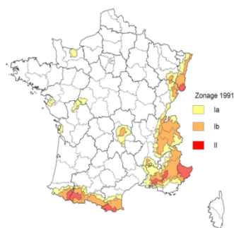
Figure 1. Ancien zonage sismique
