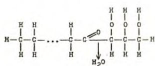
LIPIDE
