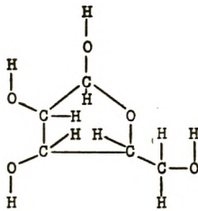
RIBOSE
