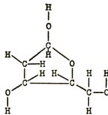
DESOXYRIBOSE
