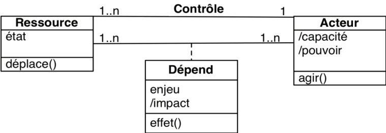
Diagramme de classe UML du formalisme SocLab
