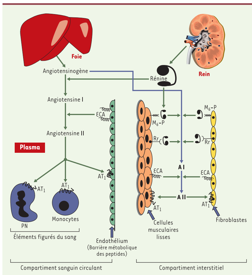
Figure 1. Compartmentation du système rénine-angiotensine. Les protéines sécrétées, rénine et angiotensinogène, diffusent dans les deux compartiments plasmatique et interstitiel, alors que les peptides, angiotensines I et II, sont métabolisés dans le compartiment où ils ont été produits. M6-P: récepteur de faible affinité du mannose 6-phosphate; Rr: récepteur de forte affinité de la rénine; ECA: enzyme de conversion de l'angiotensine; AT1: récepteur de type 1 de l'angiotensine II; PN: polynucléaire.
