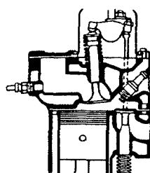
Moteur à soupapes mixtes
