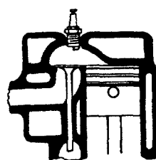
Moteur à soupapes latérales
