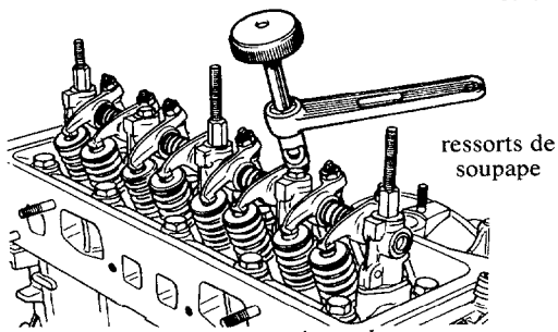
Rampe de culbuteurs montée sur le dessus de la culasse d'un moteur à quatre cylindres
