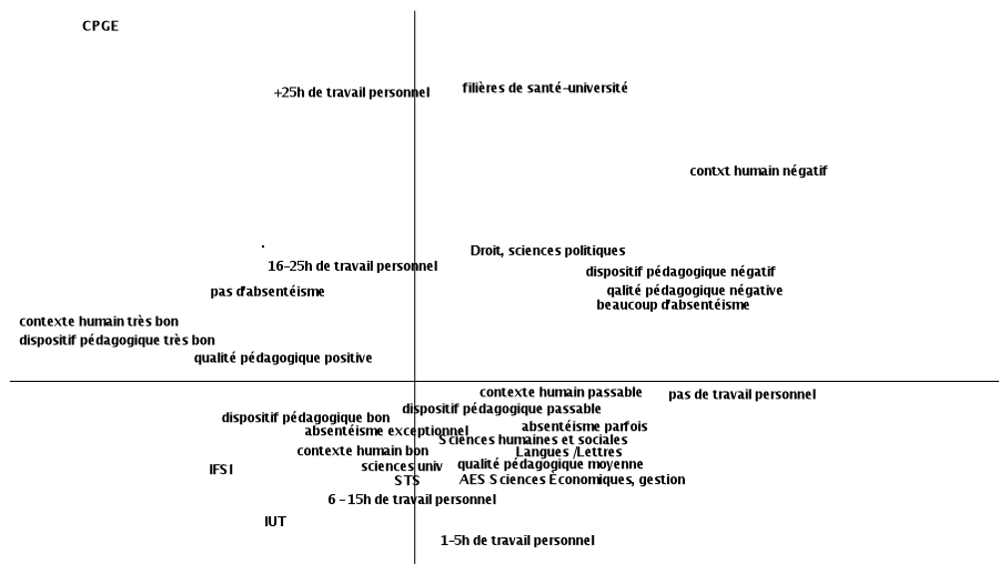
Figure 3. Schéma factoriel (facteurs 1 et 2) : L'investissement studieux des étudiants selon la filière d'études et le niveau de satisfaction de l'environnement d'études (facteur 1 = 19,4% et facteur 2 = 12,6%)
