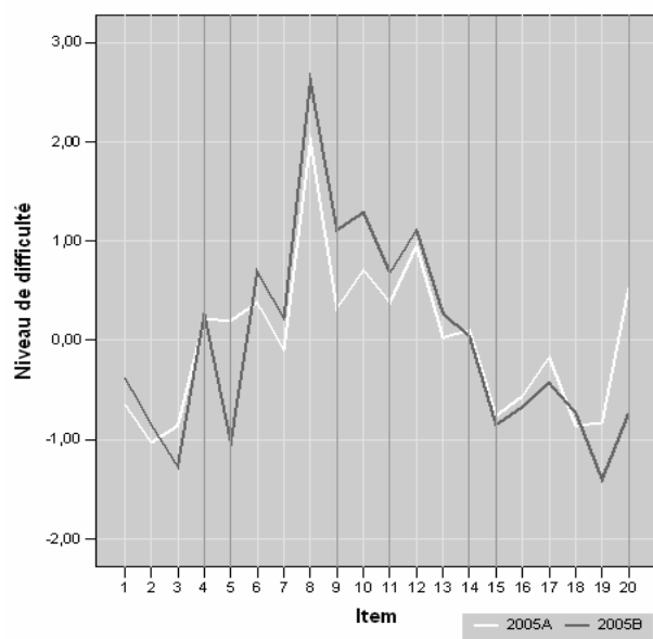
Figure 2. Position relative de la mesure estimée par le modèle pour le niveau d'endossement des items pour les versions A et B des questionnaires 2004 et 2005
