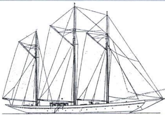
Plan de voilure du yacht Xafira qui deviendra plus tard l' Oiseau blanc , revue Le Yacht , 10 septembre 1927.
