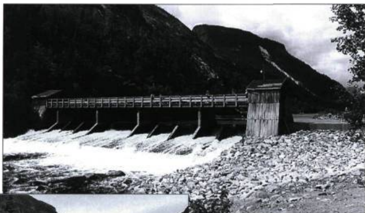
Le barrage des Hautes Gorges. En haut : après la réfection en 1997.
