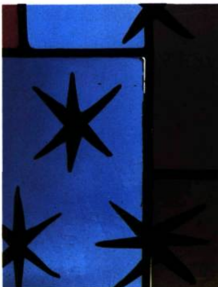
Le jour entre les plombs et les verres est la conséquence d'un mauvais travail d'assemblage. (photo: Jean-Guy Kérourac)
