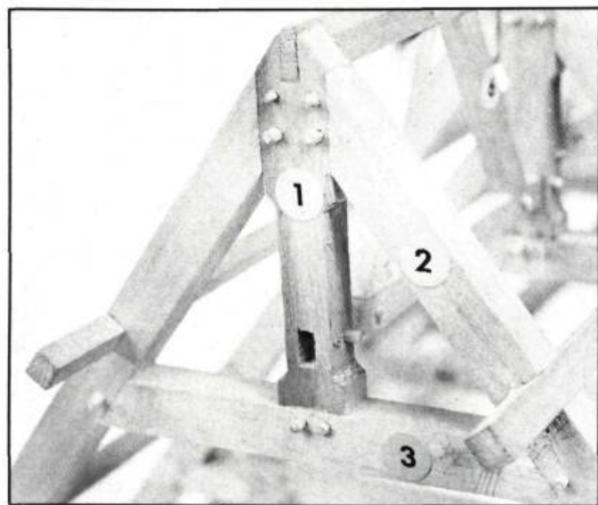
Détail de la maquette de la charpente du Manoir Mauvide-Genest réalisée par Denis Tétrault. Les numéros indiquent les pièces de la charpente: 1. le poinçon; 2. le chevron; 3. le faux-entrait. Les lignes parallèles sur le faux-entrait reproduisent celles tracées par le charpentier du côté ouest au XVIII e siècle. Il s'agit ici de chiffre romain puisque la forme suivante, non visible sur la photo, est marquée d'un V. (photo: S.A.V., Université Laval)
