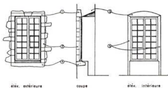
élev. extérieure
