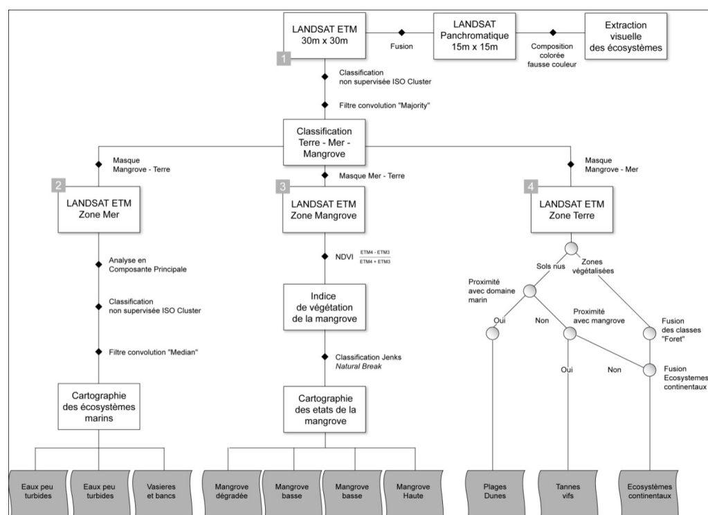
Figure 4. Schéma de la chaine de traitements pour l'extraction des écosystèmes marins et côtiers
