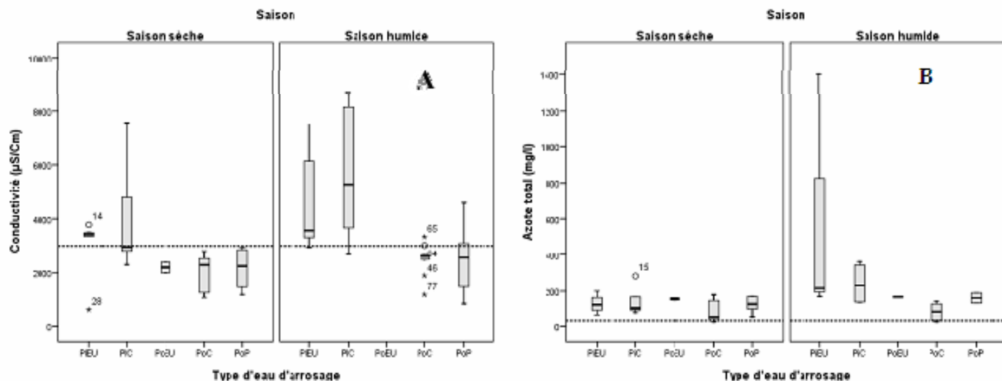
Figure 4. Variation saisonnière des paramètres chimiques des eaux d'arrosage en 2008.
