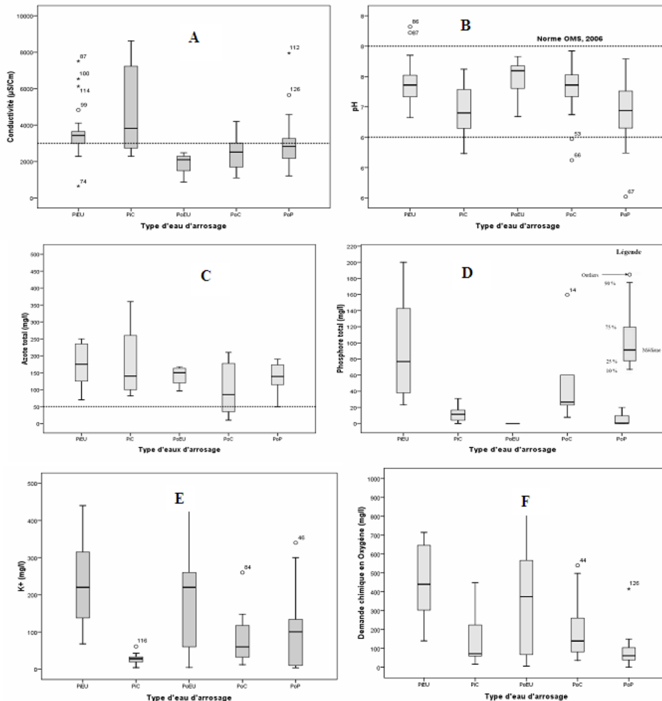
Figure 3. Caractéristiques chimiques des eaux d'arrosage.
