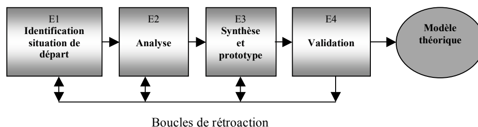
Figure 1. La stratégie générale de l'anasynthèse pour développer un modèle théorique
