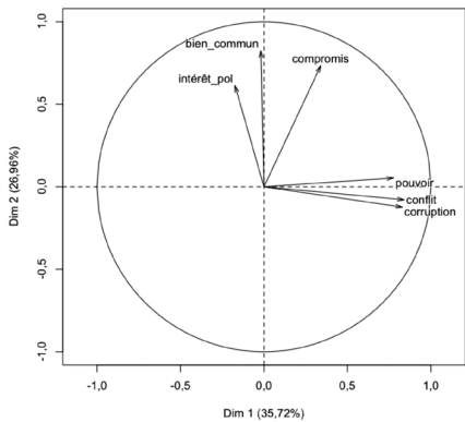
GRAPHIQUE 2 Analyse en composantes principales (les variables)
