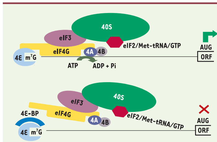
Figure 1. Contrôle de l'initiation de la traduction par 4E-BP. La fixation du complexe eIF4F (eIF4E, eIF4G et eIF4A) à la coiffe de l'ARNm à traduire et à la sous-unité ribosomique 40S engendre un balayage du messager qui permet la localisation du codon d'initiation AUG. L'interaction de 4E-BP avec eIF4E empêche l'interaction entre eIF4E et eIF4G et, par conséquent, la formation du complexe eIF4F. Pour leur part, eIF4A et eIF4B agissent, en tant que facteurs « accessoires », en dénaturant les structures secondaires de l'ARNm. Sous sa forme liée au GTP, eIF2 interagit avec les nucléotides guanines et l'ARN de transfert méthionine (met-tARNi). Le complexe ternaire ainsi formé (eIF2-GTP-met-tARNi) se lie à la sous-unité ribosomique 40S. C'est alors l'anticodon de ce met-tARNi qui reconnaît le codon d'initiation présent dans l'ARNm. ORF : origin of replication .
