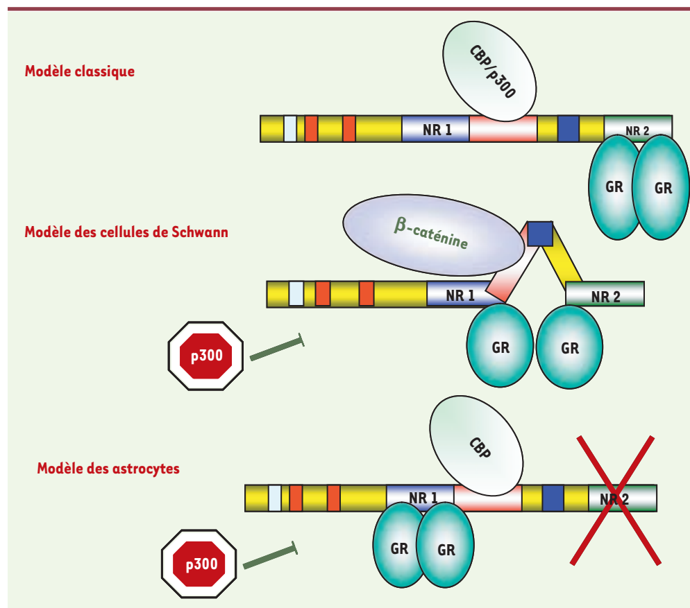
Figure 2. Modèles d'assemblage entre le GR, SRC-1a et CBP ou p300. Dans le système classique, le GR interagit exclusivement avec le NR2 en position carboxyterminale de SRC-1a, et CBP ou p300 interagissent avec la partie centrale de la protéine. Dans les cellules de Schwann, le GR interagit indifféremment avec le NR1 ou le NR2 de SRC-1a, ce qui provoque un changement de conformation de la protéine et le recrutement de la \beta -caténine à la place de la CBP ; p300 agit dans ce cas comme un corépresseur grâce à son activité histone acétyltransférase qui doit probablement acétyler une protéine du complexe transcriptionnel du GR. Dans le cas des astrocytes, le GR interagit exclusivement avec le NR1, le NR2 étant dans ce cas un domaine d'exclusion. CBP se positionne au niveau du domaine central et p300 est un corépresseur.
