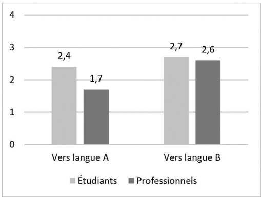
FIGURE 3 Notes moyennes pour les deux groupes de traducteurs
