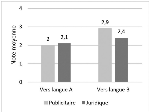
FIGURE 2 Notes moyennes pour les deux types de textes
