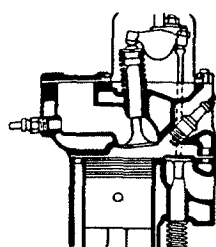
Moteur à soupapes mixtes
