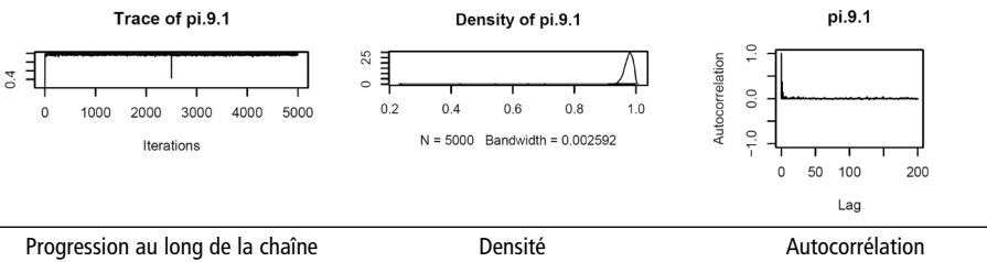
Figure 3. Exemple de graphiques montrant la convergence d’un paramètre \pi .
