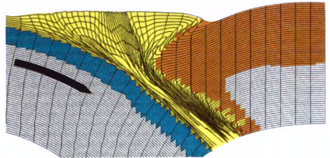
iv) Mode C: Pro-Wedge and Conduit
