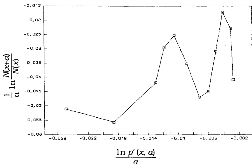
FIGURE 6 — Ajustement des décès féminins de Centrafrique par la méthode de Salhi
