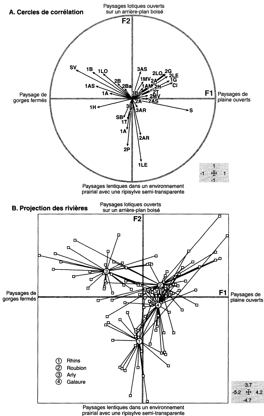
Figure 4 Cercles de corrélation, projection des rivières et projection des stations sur les plans F1 - F2 et de l'analyse en composantes principales normés
