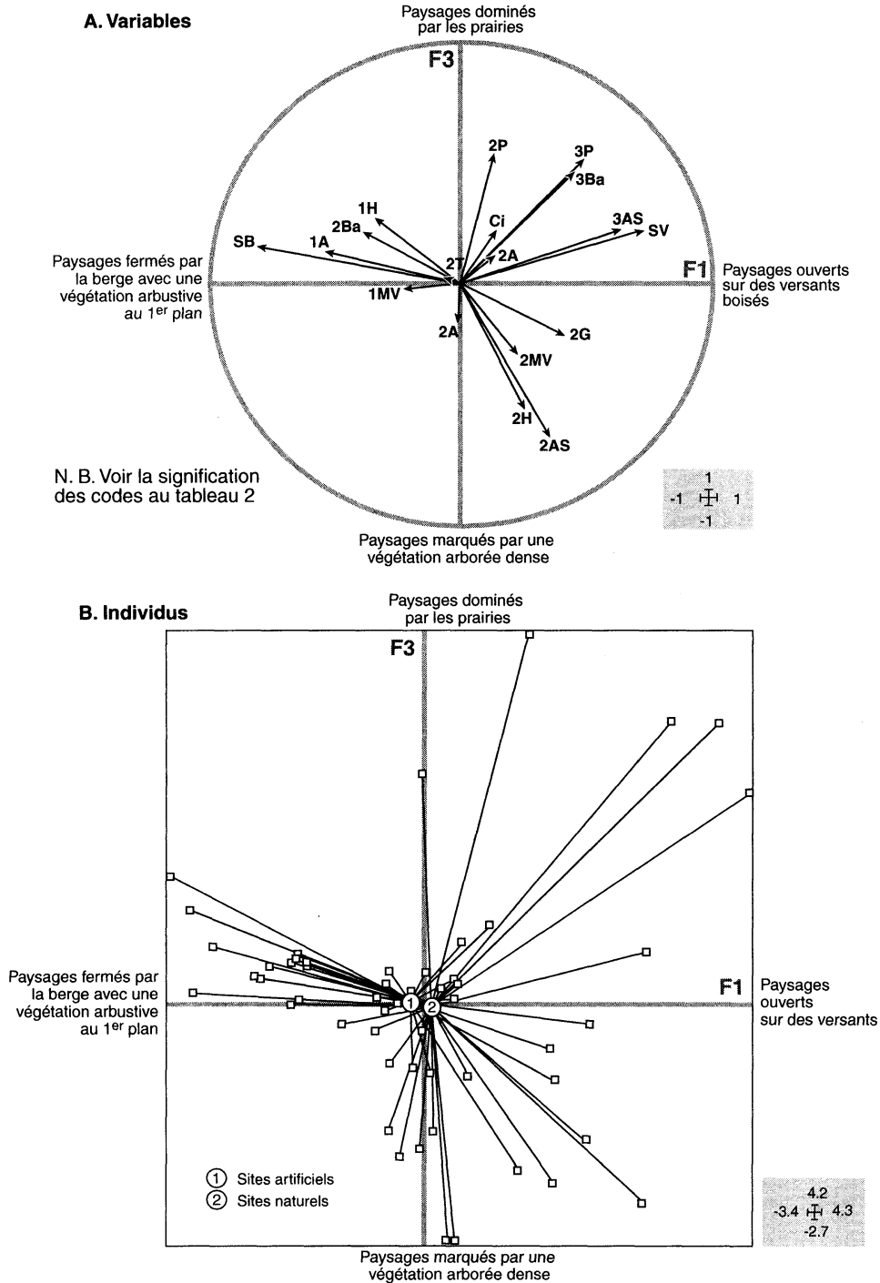
Figure 6 Projection des variables et des individus sur le plan factoriel F1F3 de l'ACPn
