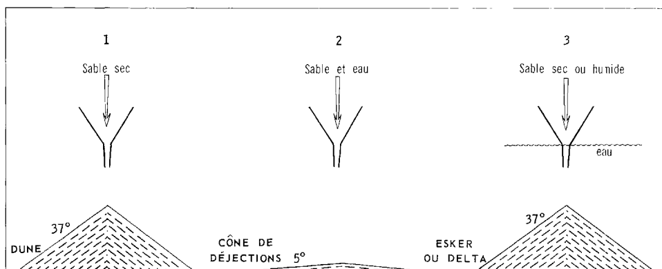
Figure 6 Expérience de sédimentation.
