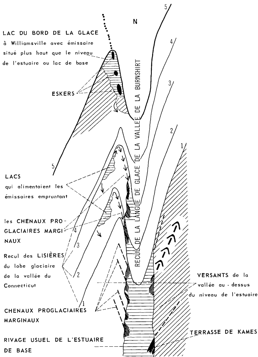
Figure 15 Présentation schématique de plusieurs lisières de gace successives montrant comment eskers et terrasses de kames se formaient d'ordinaire au niveau d'un estuaire de vallée, mais parfois aussi étaient formés au niveau de lacs du bord de la glace à des altitudes plus fortes.
