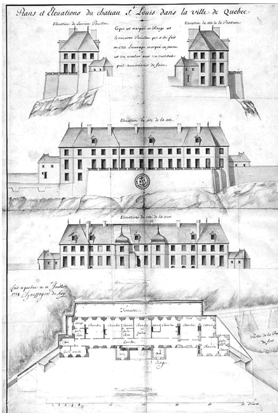
Plans et élévations du château Saint-Louis en 1724 par Gaspard-Joseph Chaussegros de Léry. ( https://fr.wikipedia.org/wiki/Château_Saint-Louis#/media/File:Plans_et_elevations_du_chateau_Saint-Louis_par_Chaussegros_de_Lery.jpg ).
