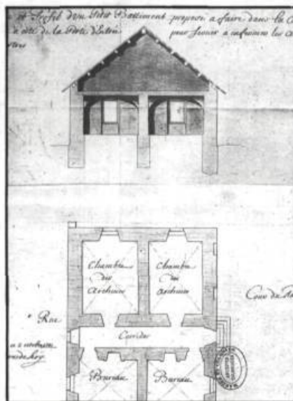
Plan et profil d'un futur dépôt d'archives à être construit dans la Cour du Palais de l'intendant. Chaussegros de Léry, Québec, 2 octobre 1731.
