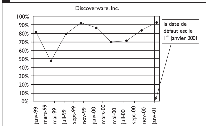
FIGURE 1 ÉVOLUTION TRIMESTRIELLE DES PROBABILITÉS DE DÉFAUT (PD) PRÉDITES POUR LES FIRMES DISCOVER- WARE (JANVIER 1999 À JANVIER 2001) ET ALGO GROUP INC. (DE 1990 À 2004)
